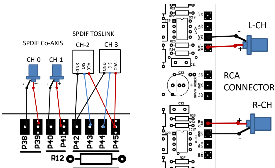
(a) 入力の接続例 (SPDIF, ANALOG)
