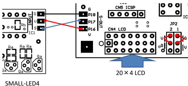
図 表示器の接続例(LCD を取り付ける場合は JP2 の設定も行います)
