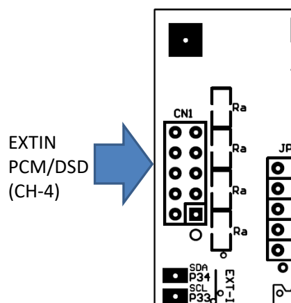
図 入出力の接続(その 2、EXTIN (PCM/DSD) 入力)
