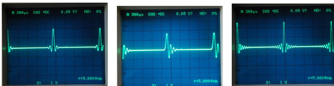
図 DAC8741 ではフィルター応答が選択可能です（パルス入力時の応答波形例）
