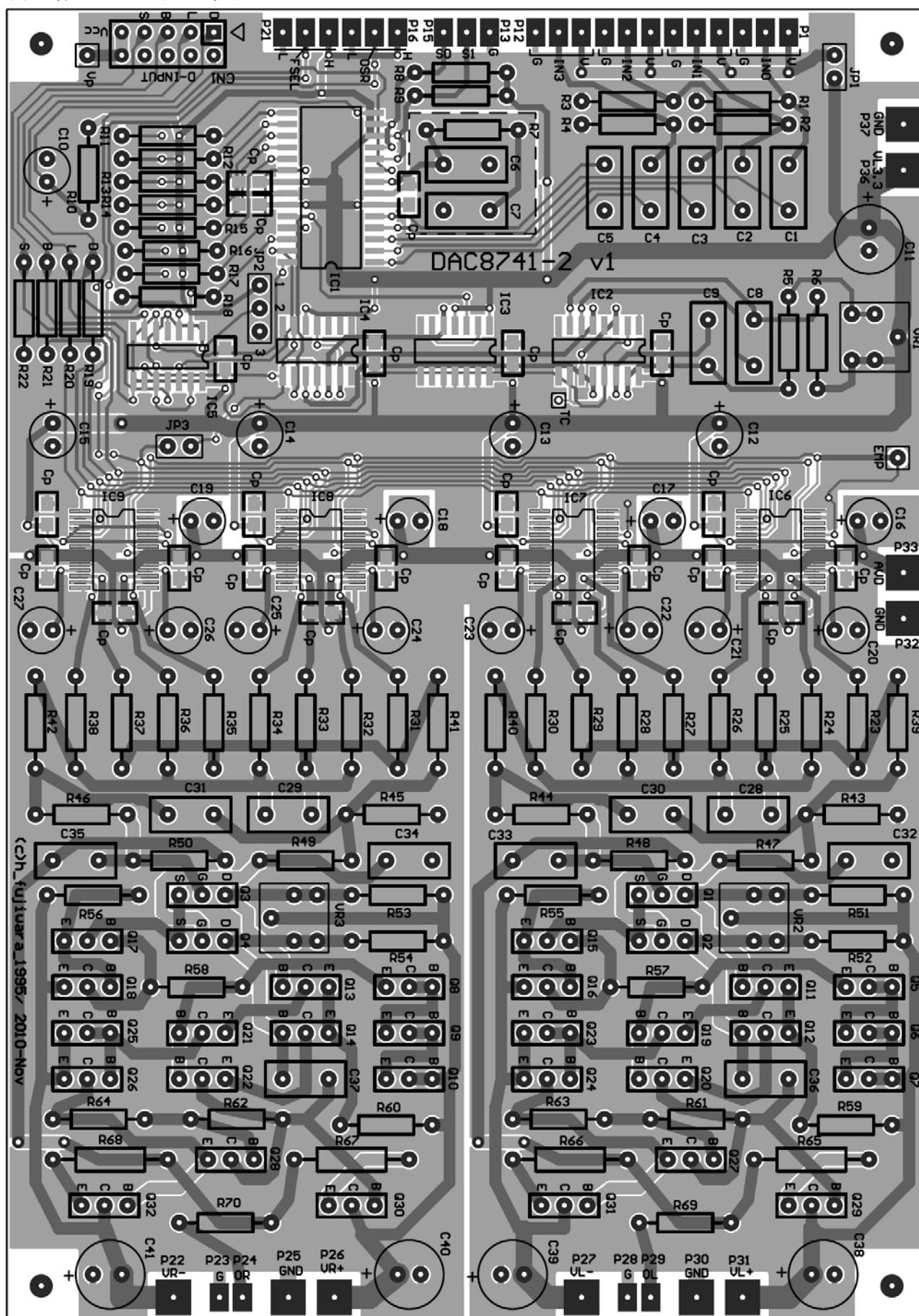
(b) 配線パターン (V1 基板)
