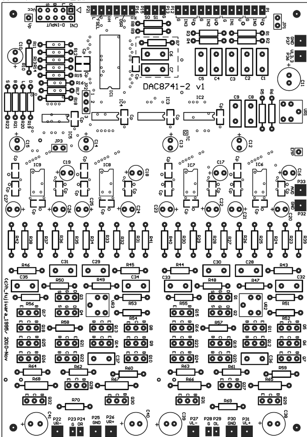
(a) シルクパターン (V1 基板)
