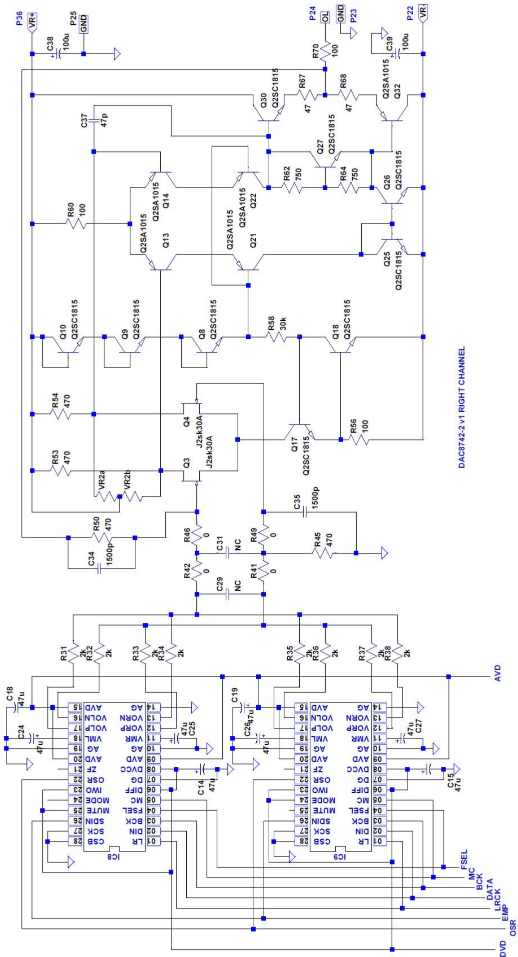
(b) DAC&アナログ部（右チャンネル） ※下図で Q27 は Q28 の間違い
