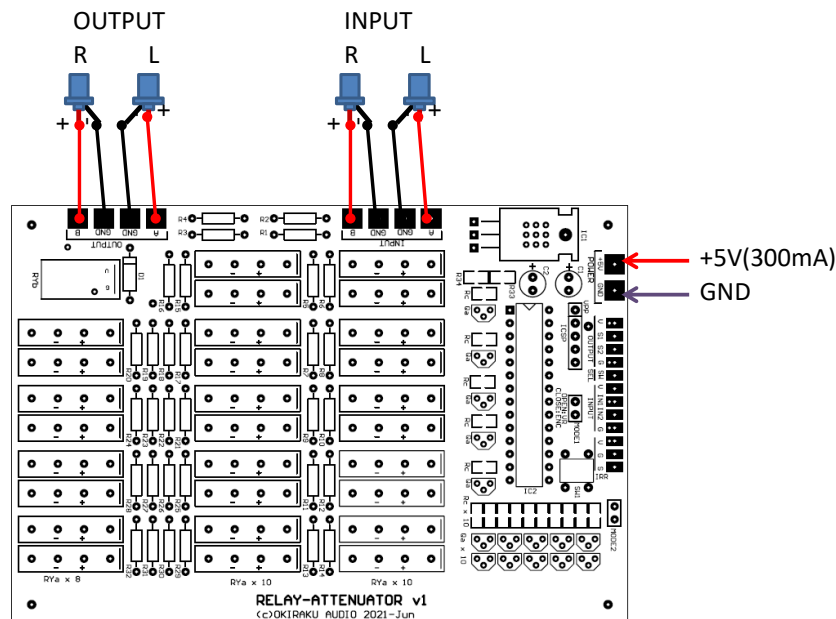
図 電源と入出力の接続例
