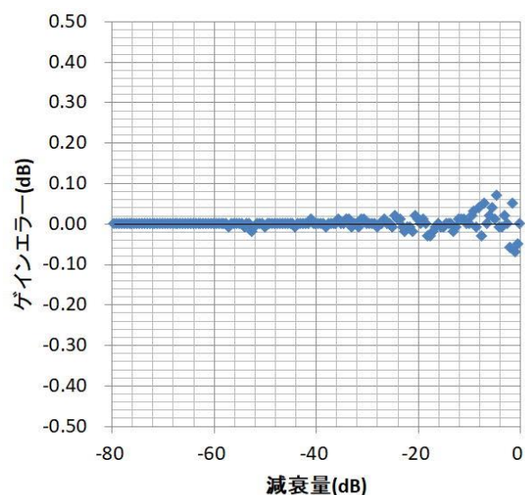
図 設定減衰量と実際の減衰量の差
